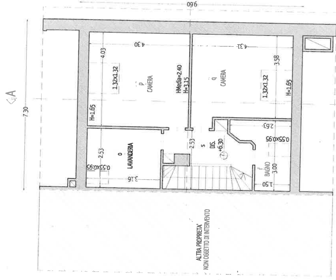
PIANO SOTTOTETTO ATTUALE SCALA 1:100 SUP. ABITAZIONE MQ=70.08
