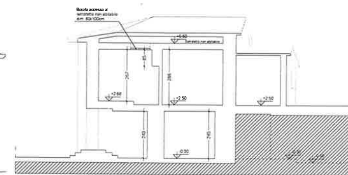
SEZIONE B-B scala 1:50
