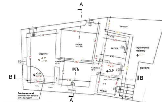
PIANO PRIMO (SDF) scala 1:50
