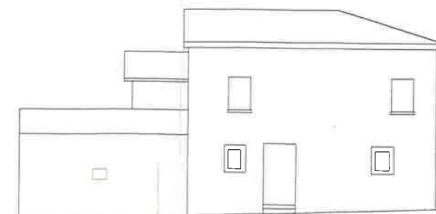
FIANCO SINISTRO scala 1:50
