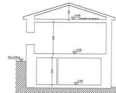
SEZIONE A-A scala 1:50
