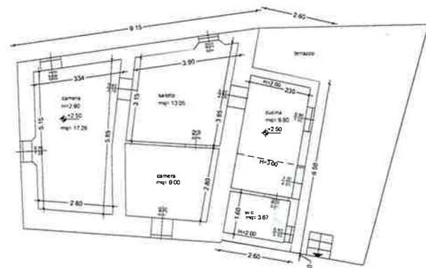
PIANO PRIMO (approvato CTE 11326) scala 1:50
