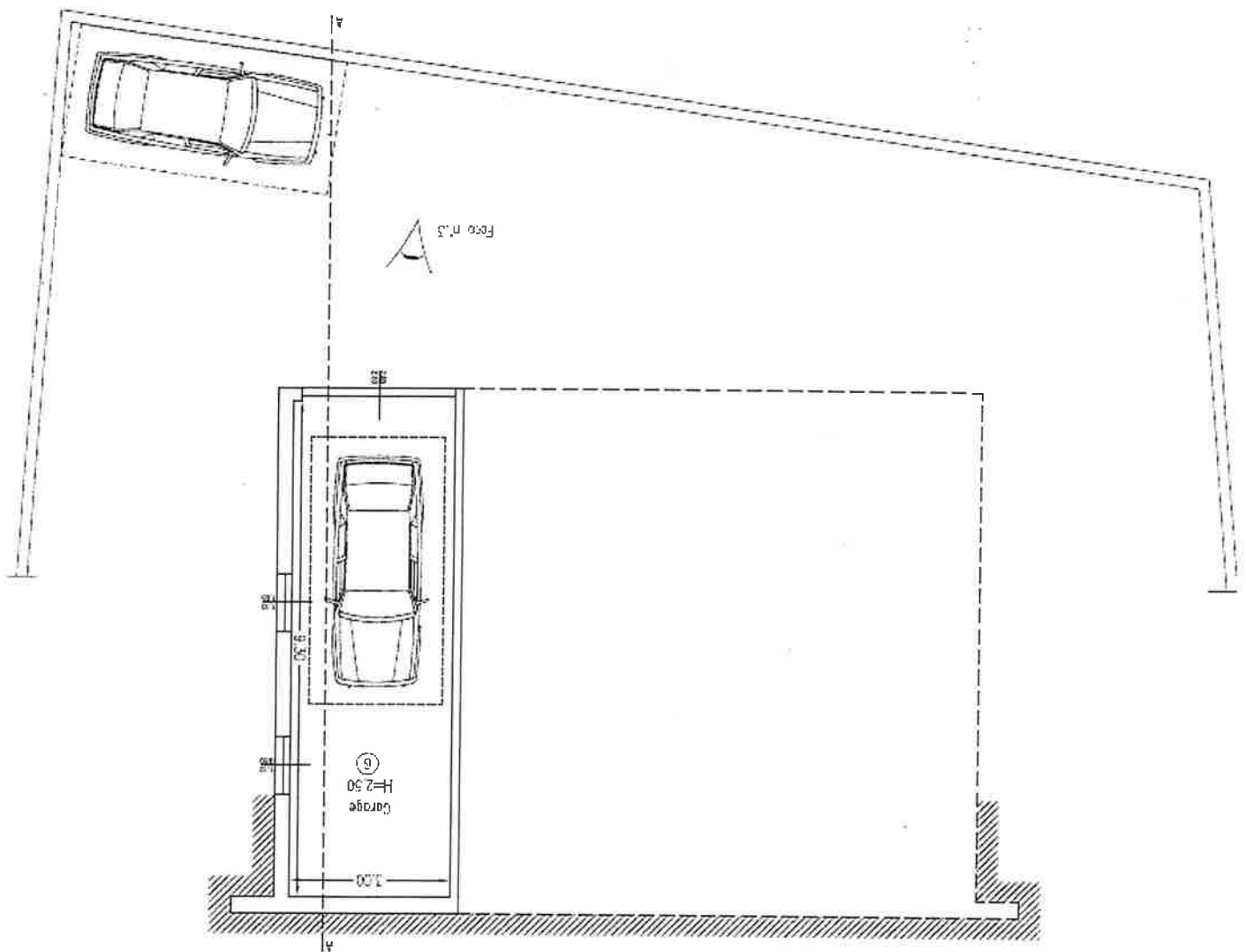
PIANTA PIANO SEMINTERRATO - Scala 1:100
